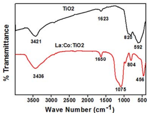
Figure 9. FT-IR Spectra of (a) \text{TiO}_2 (b) \text{La:Co:TiO}_2 .
