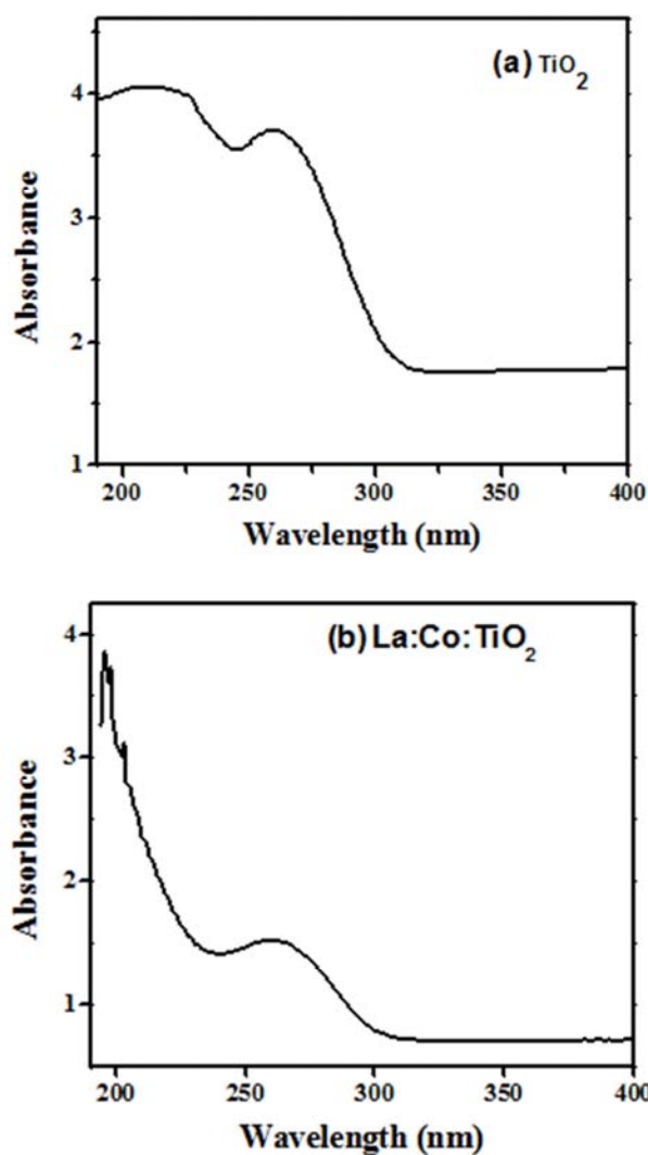
Figure 7. UV- Vis. Spectra of (a) TiO 2 (b) La:Co:TiO 2 .
